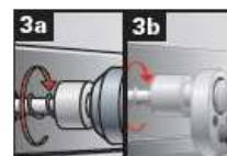
Draai de betonschroef vast met een steeksleutel (sleutelmaat SW 15). Neem de maximale aandraaimomenten in acht.
