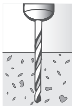
1) Markeer boorpositie en boor (Ø 16 mm, min. 100 mm diep)
