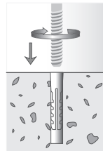
3) Plaats de kluis en draai schroef M12 met sluitring in
