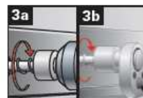
3a 3b Serrez la vis à béton avec une clé à douille (taille de clé SW 15). Respectez les couples de serrage maximum.
