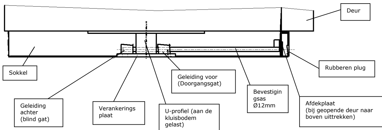
Afbeelding 9. Zijaanzicht verankeringsysteem
