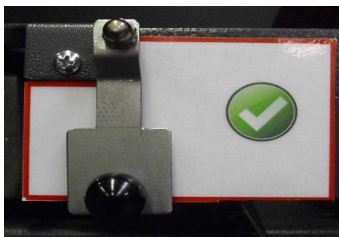
Terugloopblokkering vrij (normale positie)
