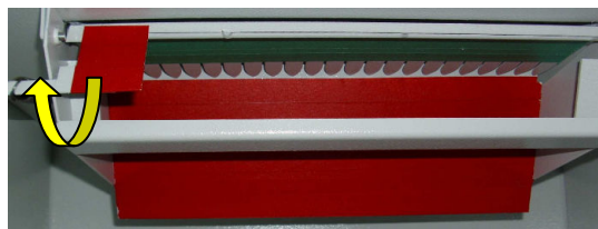
Dispositif anti-retour verrouillé (déclenché)
